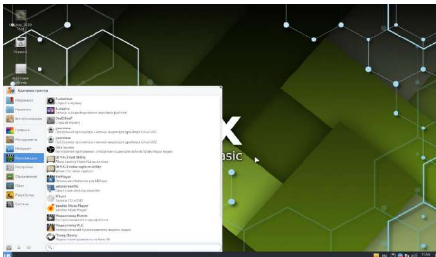
Рисунок 40. Программы мультимедиа
