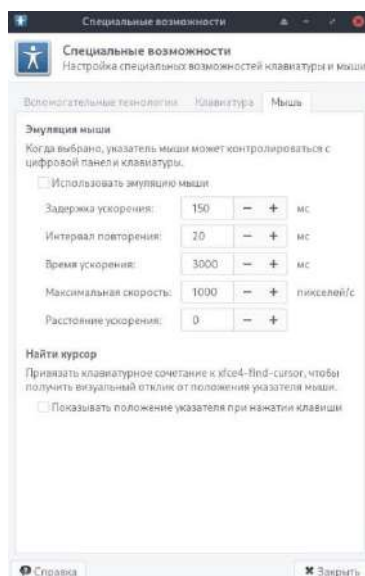
Рисунок 29. Специальные возможности
