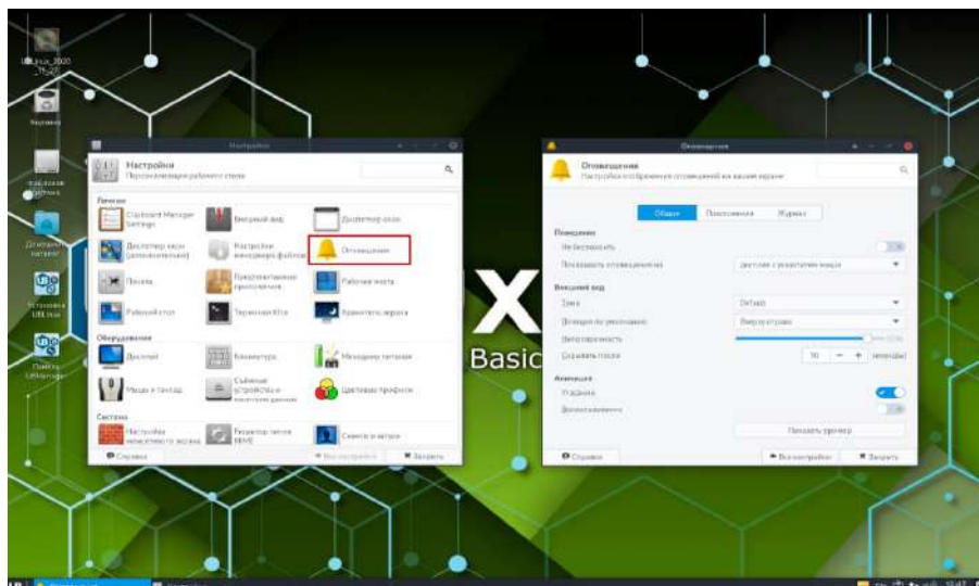
Рисунок 13. Окно «Оповещения»
