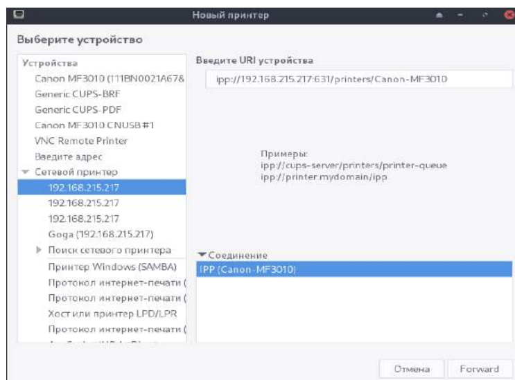
Рисунок 25. Окно «Новый принтер»
