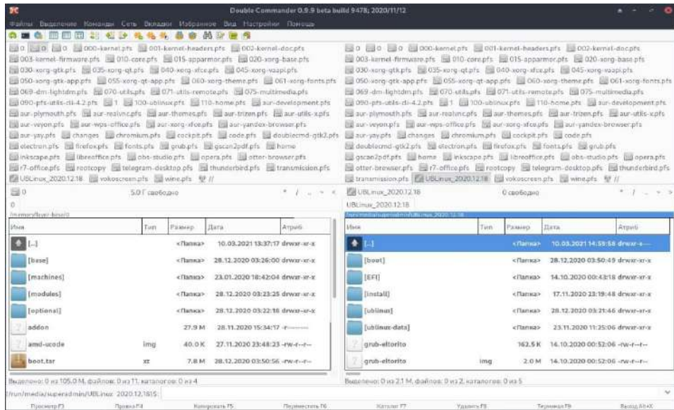
Рисунок 37. Double Commander
