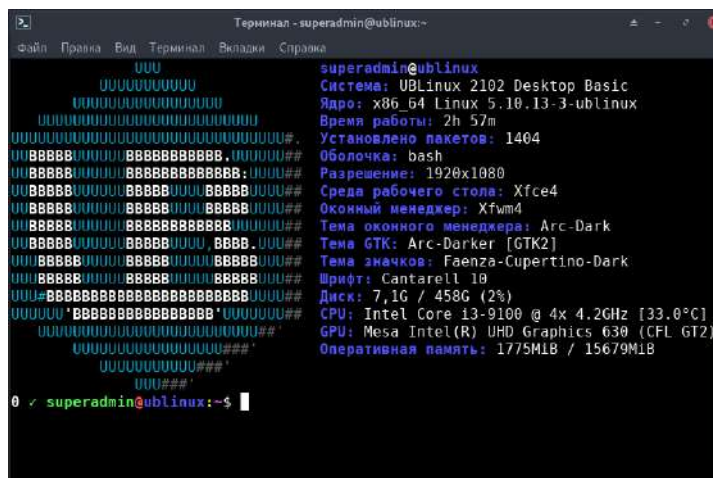
Рисунок 30. Открытый терминал
